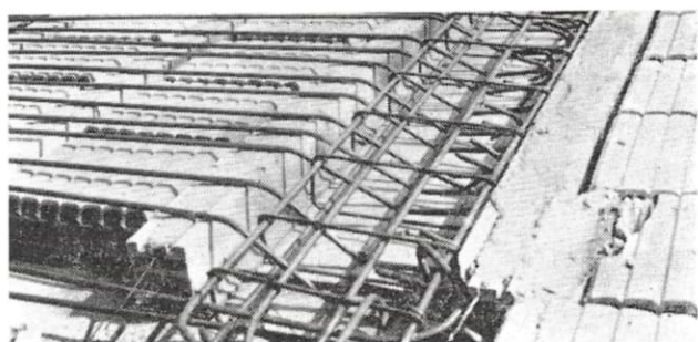
Armatura in procinto di gettata - Geom. Pagni e Guerri
